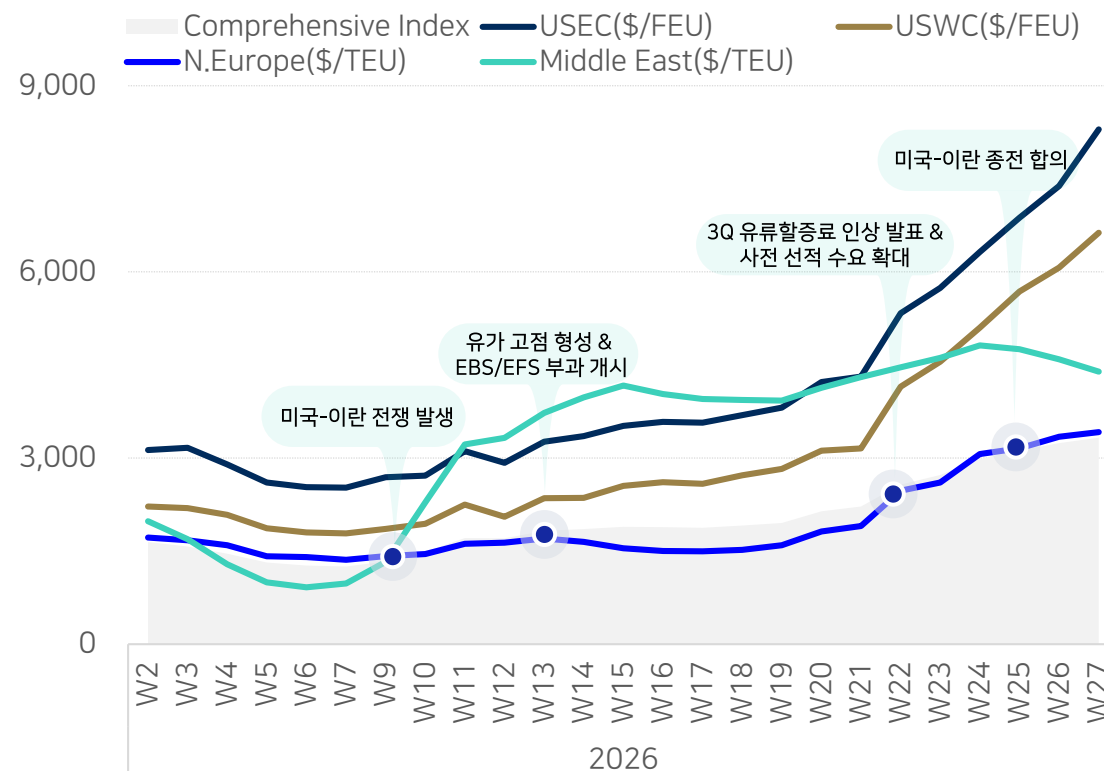
['26년 주요 항로 SCFI 트렌드]
